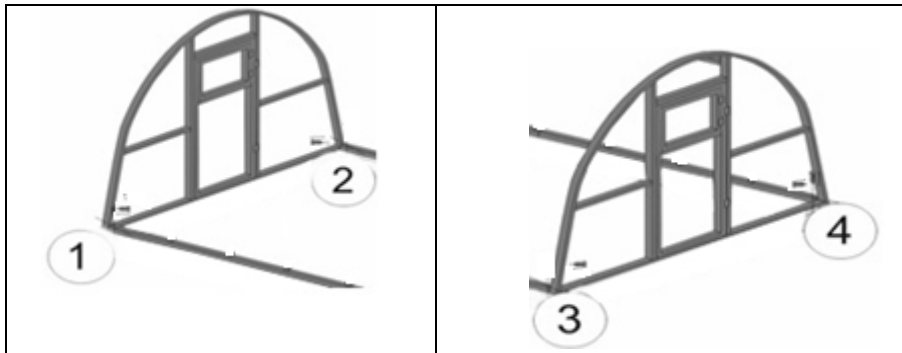
Pav. 9. Sujungimo vietos naudojant savisriegius varžtus (pozicija Nr. 1, 2, 3, 4). Jei šiltnamio tvirtinamas prie pamato, tvirtinimui naudojami savisriegiai varžtai (Pav. 10).
